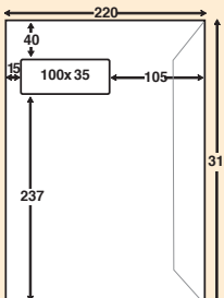
V2-Tverrstilt vindu E4
