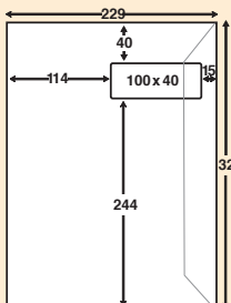
H2-Tverrstilt vindu C4
