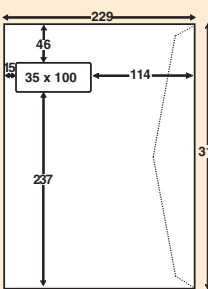
Vindu nr. 19. C4M
