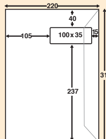
H2-Tverrstilt vindu E4
