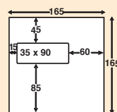
Vindu nr. 11. 165 x 165 høyt vindu venstre
