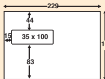
Vindu nr. 16. C5 høyt vindu venstre
