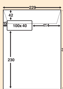
Vindu nr. 18. EC4
