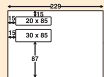
Vindu nr. 33/2. C5 2 vinduer
